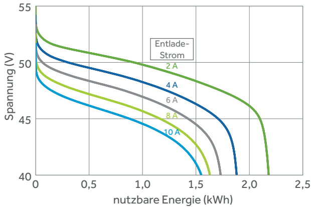
Spannung / nutzbare Energie (nach 10-stündiger Ladezeit)
