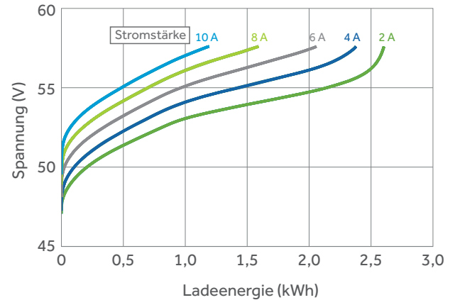
Spannung / Ladeenergie
